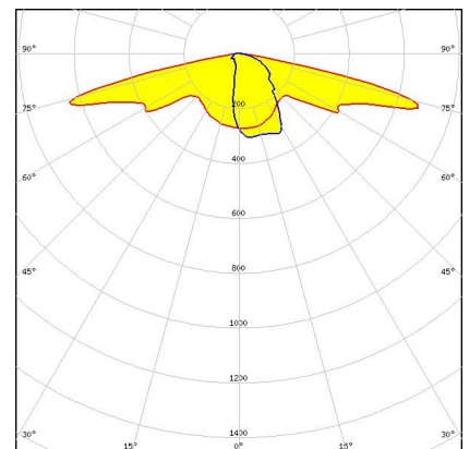
C14517_STRADA-2X2-DWC-PC
