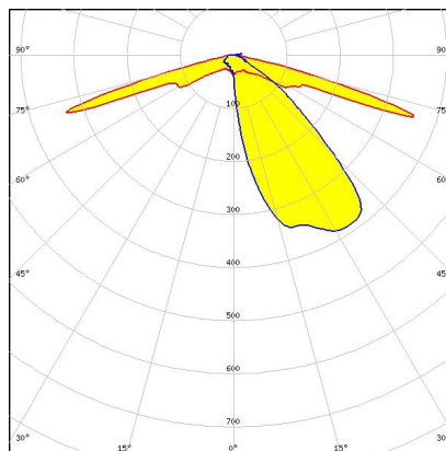
C16795_STRADA-2X2-T2-M-PC
