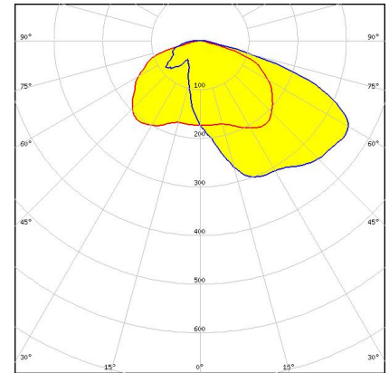
C13805_STRADA-2X2-T4
