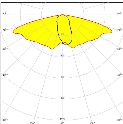
C17118_STRADA-2X2-T1-M
