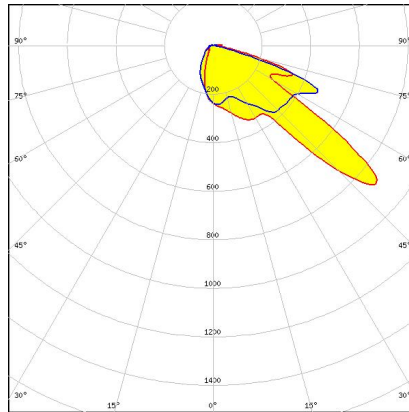
C14116_STRADA-2X2-PX
