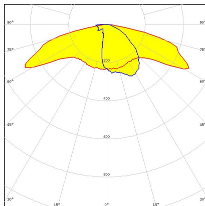
C12362_STRADA-2X2-DWC
