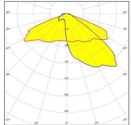
C15594_STRADA-2X2-MEW
