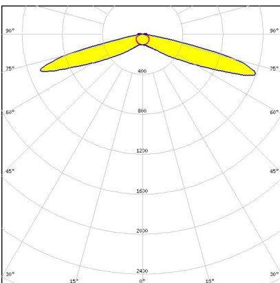
C15135_STRADA-2X2-T1
