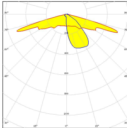
C16504_STRADA-2X2-T2-M
